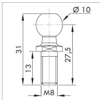
► Rotule acier Ø 10 pour cage M8 Réf. : 92990
