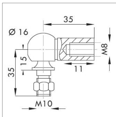
► Cage à rotule Ø 16 avec rotule M8-M10 acier Réf. : 92262-10-8
