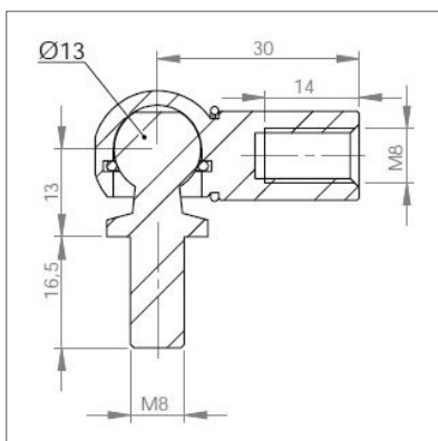
► Cage à rotule acier Ø 13 avec rotule M8 Réf. : 92262
