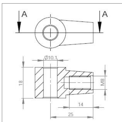
► Chape à œil Zamack 10/18 M8 Réf. : 92266
