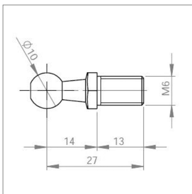
► Rotule acier Ø 10 pour cage M6 Réf. : 92989
