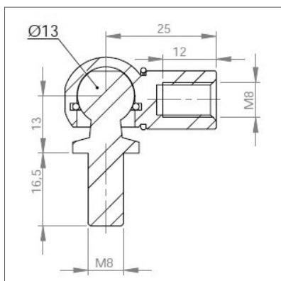
► Cage à rotule acier Ø 13 avec rotule M8 Réf. : 92265
