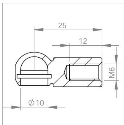
► Cage à rotule acier Ø 10 M6 Réf. : 92220
