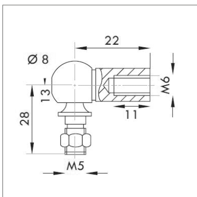
► Cage à rotule Ø 10 avec rotule acier Réf. : 92220-6-5
