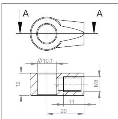
► Chape à œil Zamack 10/12 M8 Réf. : 92267
