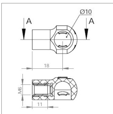
► Cage à rotule plastique Ø 10 M6 Réf. : 72421
