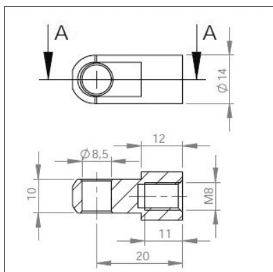
► Chape à œil Acier 8/10 M8 Réf. : HGCH8
