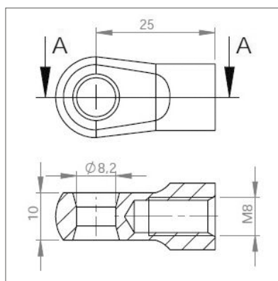
► Chape à œil Zamack 8/10 M8 Réf. : 92264
