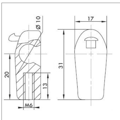
► Cage à rotule plastique Ø 10 M6 Réf. : 92722
