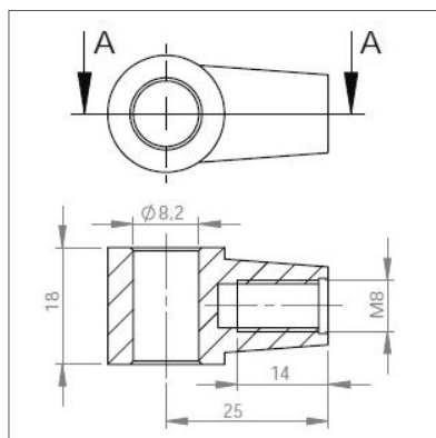
► Chape à œil Zamack 8/18 M8 Réf. : 92260
