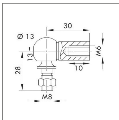
► Cage à rotule Ø 13 avec rotule acier Réf. : 92220-13E
