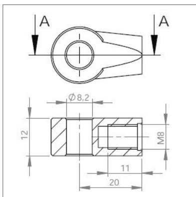
► Chape à œil Zamack 8/12 M8 Réf. : 92261
