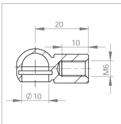
► Cage à rotule Acier Ø 10 M6 Réf. : 92221
