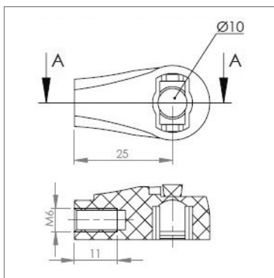
► Cage à rotule plastique Ø 10 M6 Réf. : 92720
